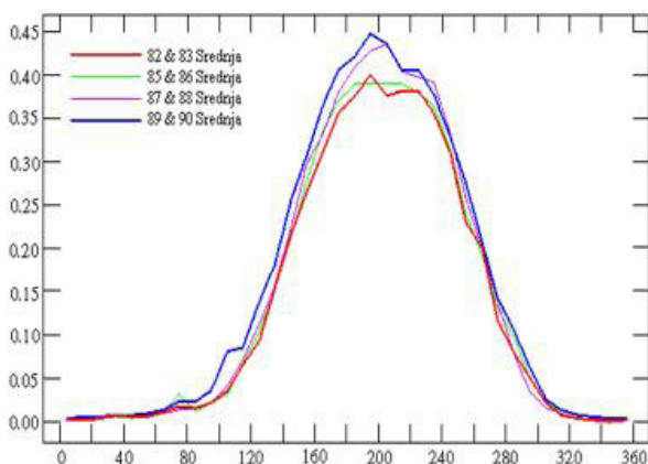
Fig. 3.4.1.3.2. Spatial average NDVI (>45° N)
